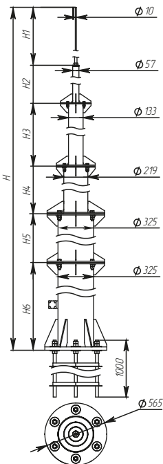
Рисунок / Figure / Сурет 14 – Мачты высотой 27000, 28500, 30000 мм / Air-termination mast 27000, 28500, 30000 mm high / Биіктірі 27000, 28500, 30000 мм діңгектер
