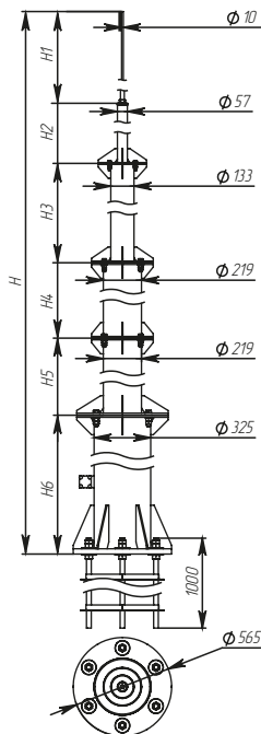
Рисунок / Figure / Сурет 13 – Мачта высотой 25500 мм / Air-termination mast 25500 mm high / Биіктірі 25500 мм діңгек
